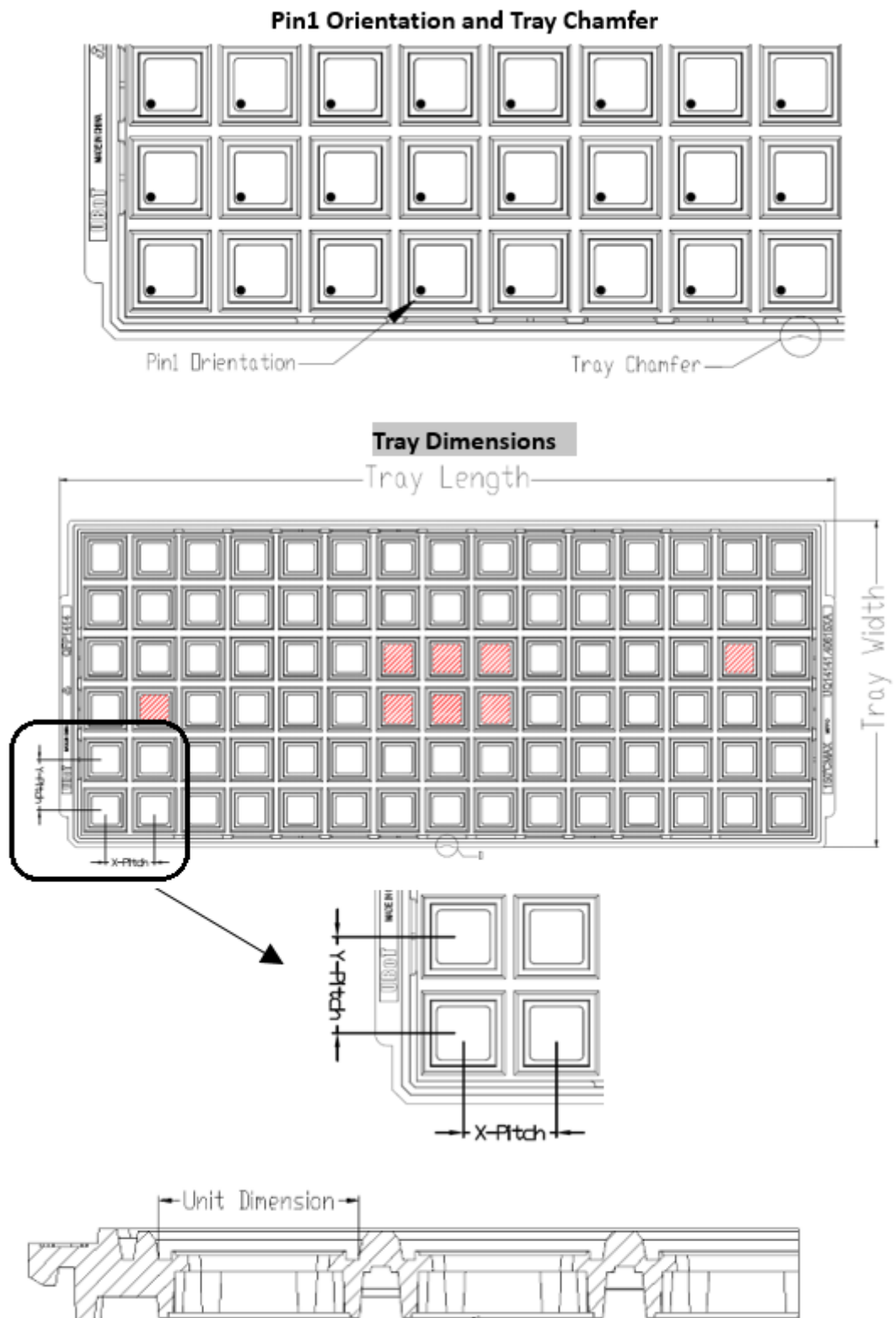
图 23 托盘包装示意图
