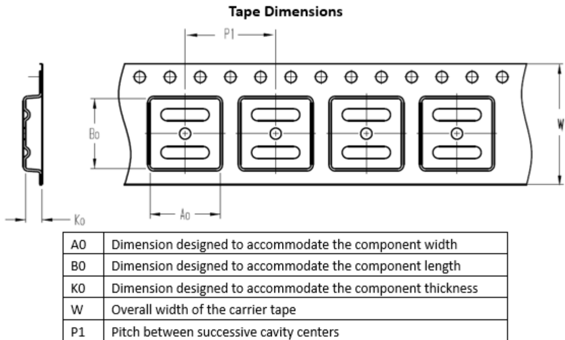
图 22 带状包装规格图
